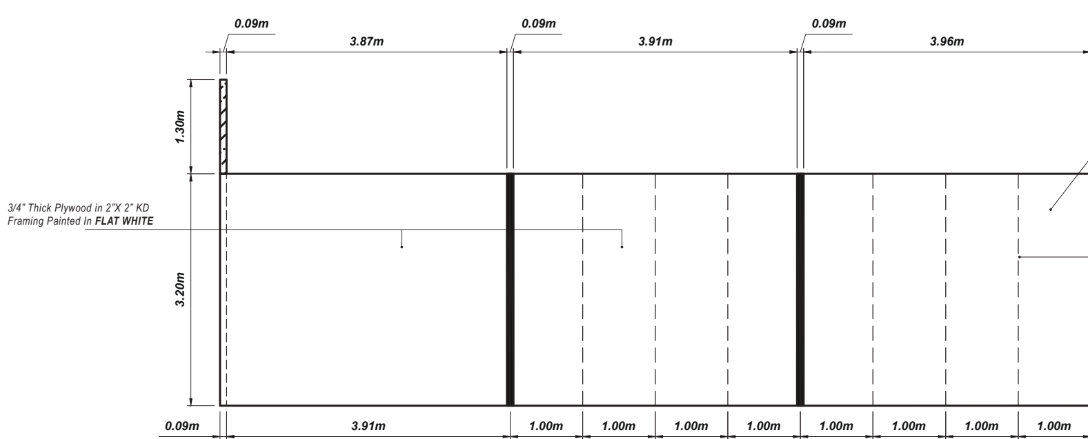
ELEVATION 1 A-2
