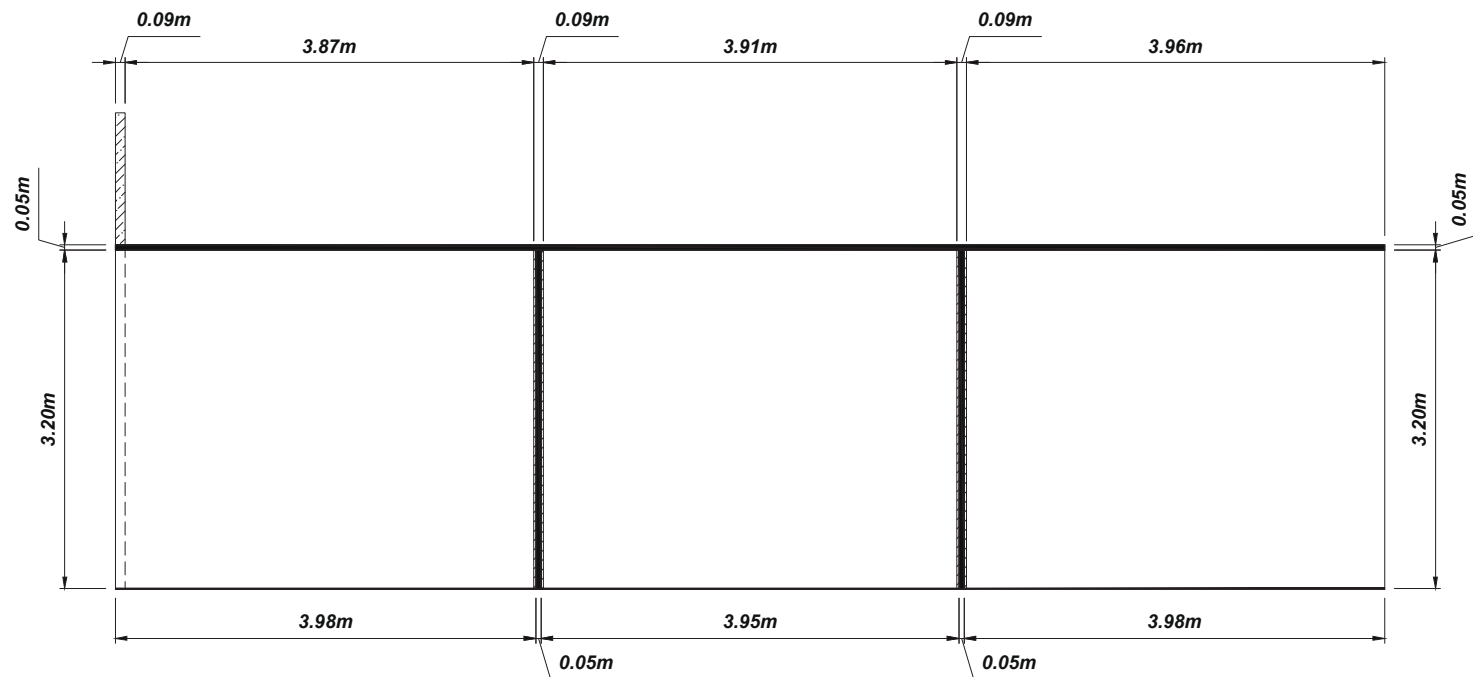
ELEVATION 2 B-2
