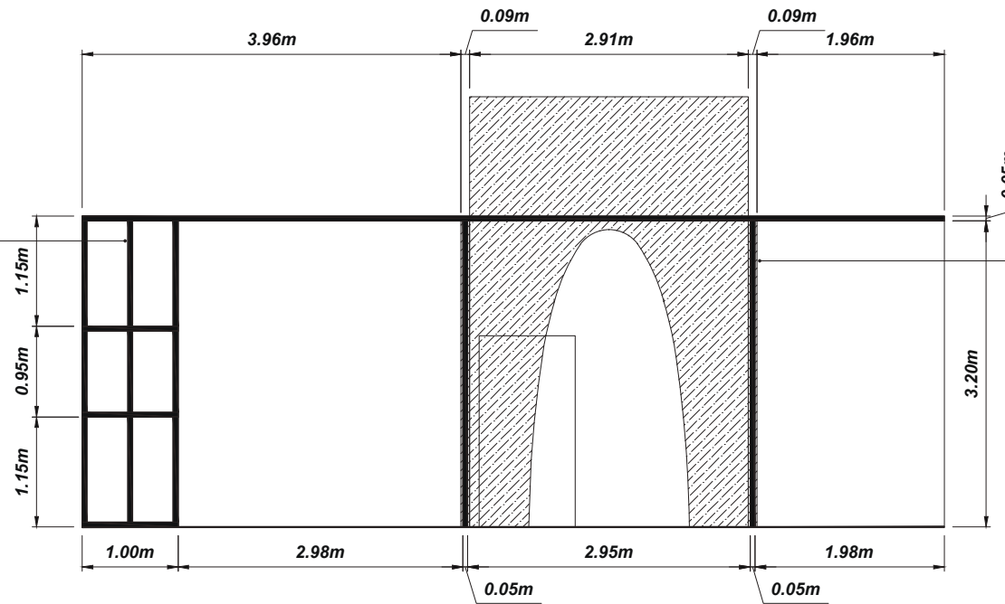
ELEVATION 2 B-3
