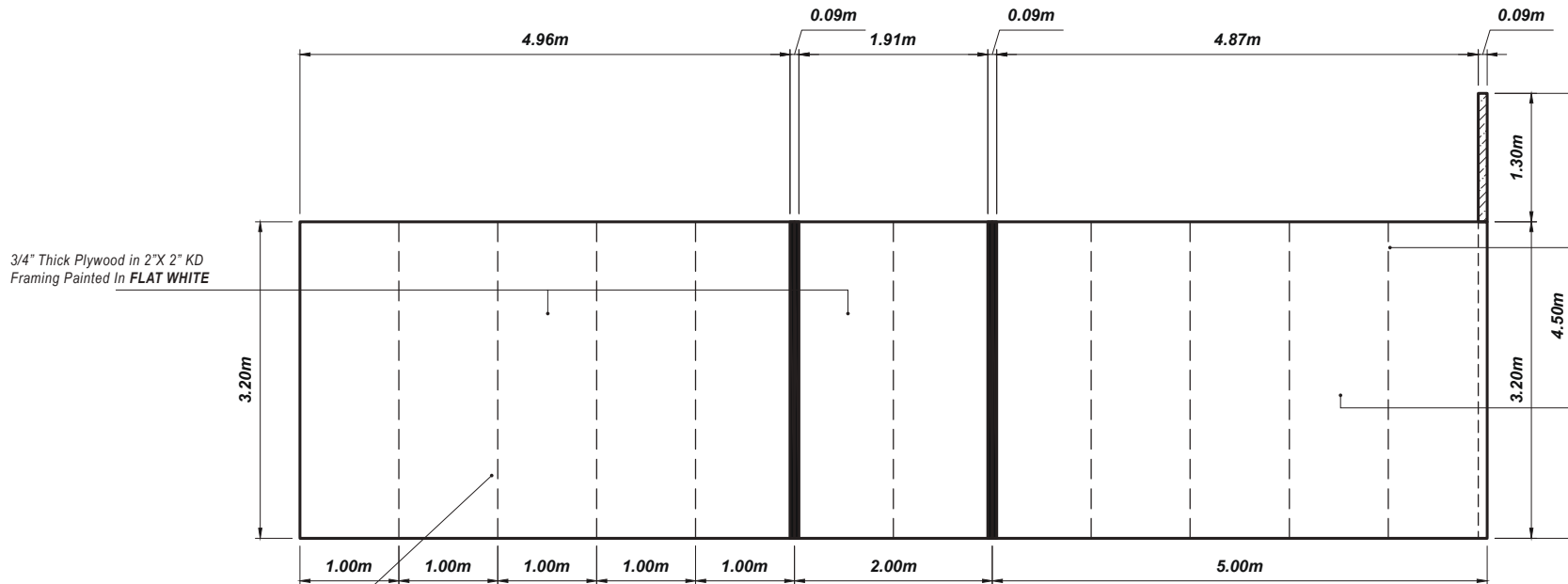
ELEVATION 1 A-1
