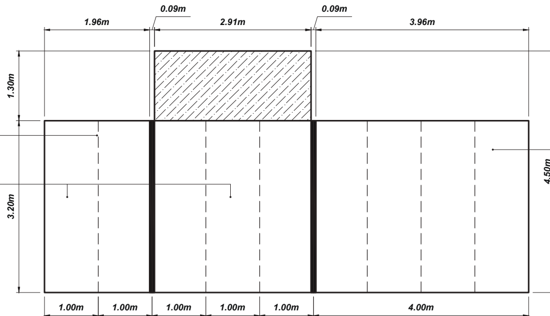
ELEVATION 1 A-4
