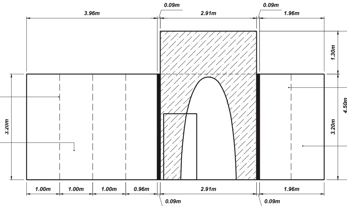
ELEVATION 1 A-3
