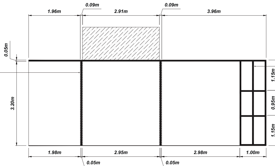
ELEVATION 2 B-4
