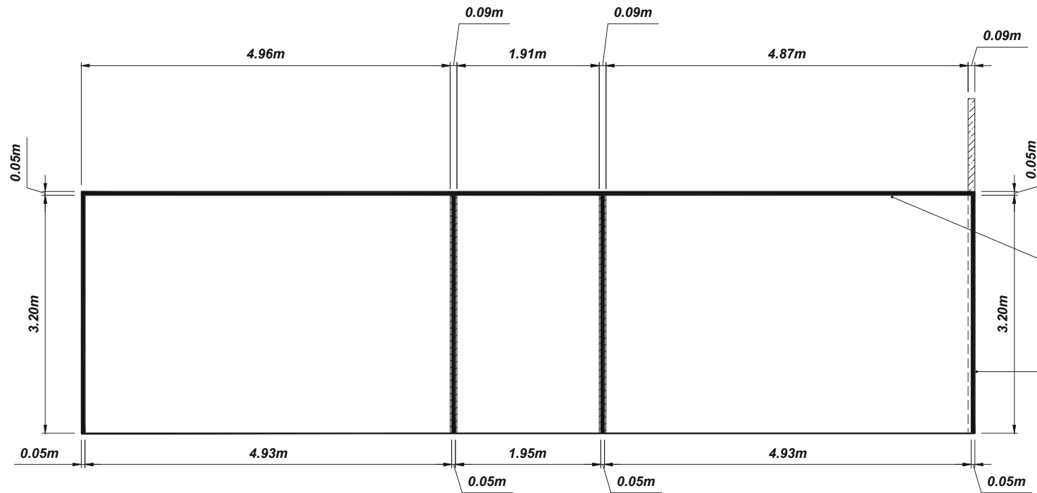
ELEVATION 2 B-1
