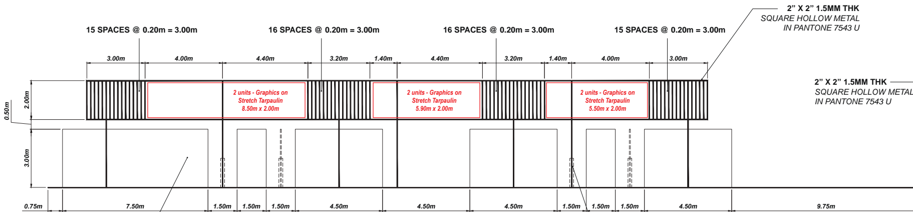
ELEVATION A3
