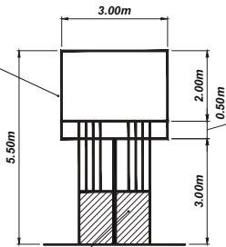
ELEVATION A4
