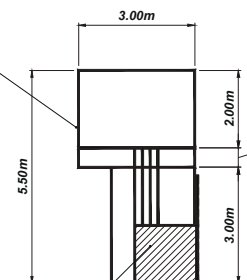
ELEVATION A2
